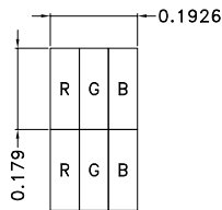
Dots Detail Scale: 100/1
