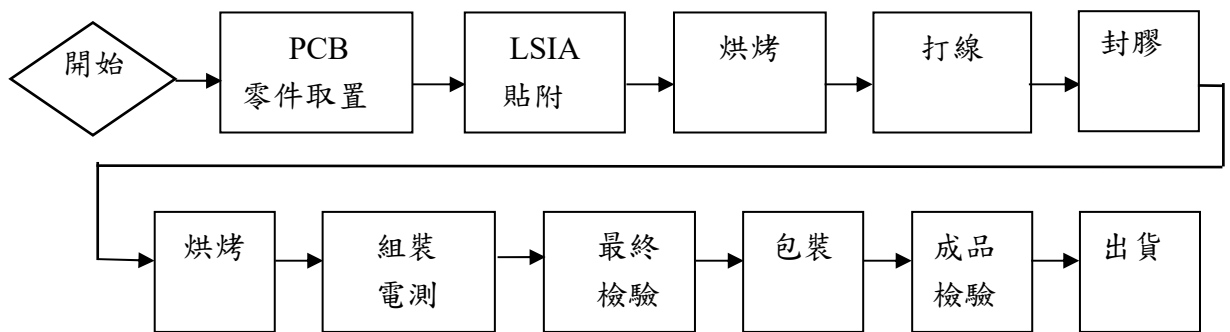
(5)COB生產流程圖
