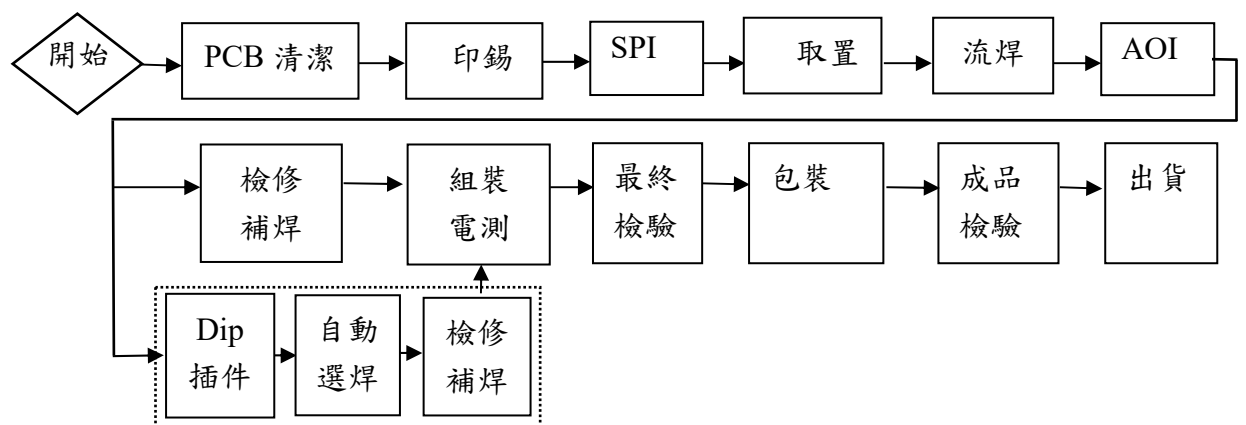
(6) SMD生產流程圖(虛線區為 Dip 自動選焊機)
