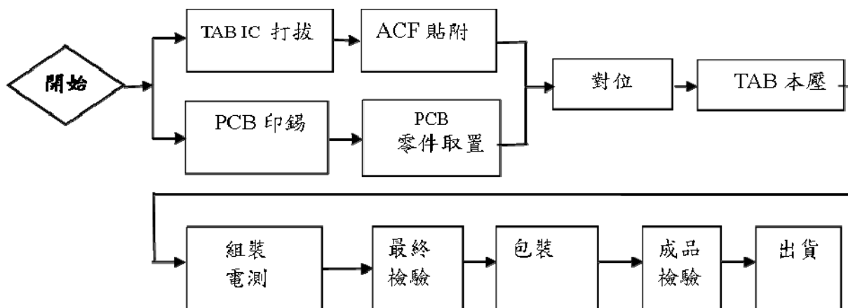
(7) TAB 生產流程圖
