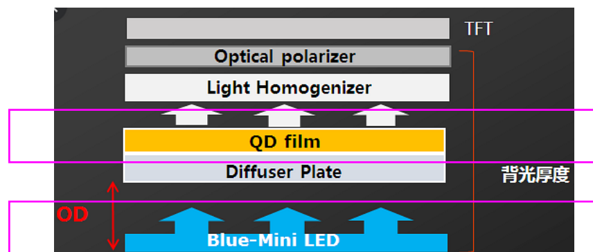
13.3" MINI LED Prototype結構
